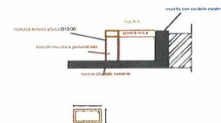
Sez. strutturale 1:100
