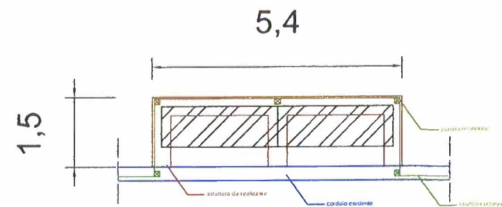
Pianta schema strutturale 1:100
